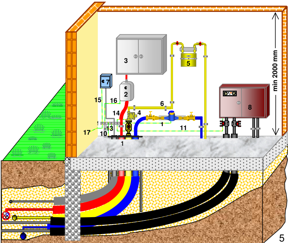
Bild 2 - Die Hausanschlusswand für \leq 4 Wohneinheiten Beispiel eines nicht unterkellerten Gebäudes
