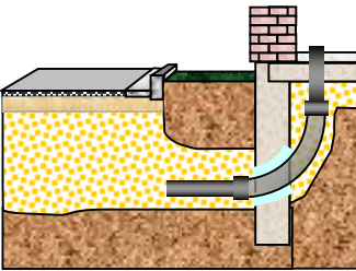
7) Hauseinführung für Häuser ohne Keller bei Einsatz eines geeigneten Kunststoffrohrbogens (in Abstimmung mit NB/WVU)
