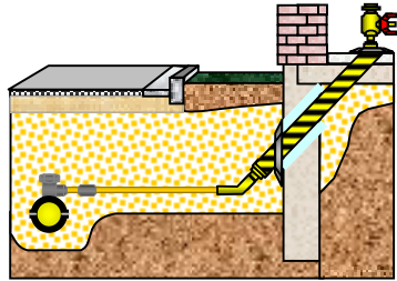
6) Hauseinführung für Häuser ohne Keller
