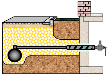
8) Hauseinführung für Häuser mit Keller
