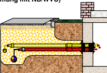
9) Mehrspartenhauseinführung für Häuser mit Keller (2/4 Medien)
