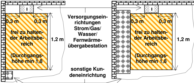
Bild 2 - Die Hausanschlusswand für \leq 4 Wohneinheiten Beispiel eines nicht unterkellerten Gebäudes
