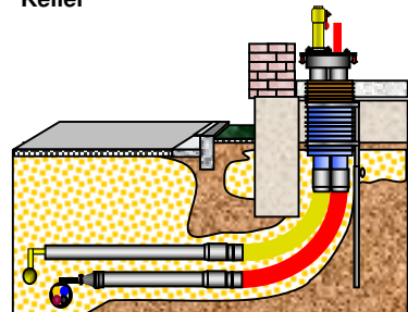
10) Mehrspartenhauseinführung für Häuser ohne Keller (2/4 Medien)
